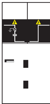
Medição de corrente e/ou de tensão com seccionadora e transições superiores por barras GBC-I (750 mm)
