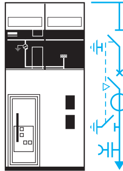
Disjuntor desconectável simples seccionamento DMVL-A (750 mm)
