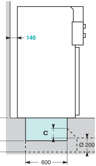
Células de 630 A Entrada ou saída frontal
