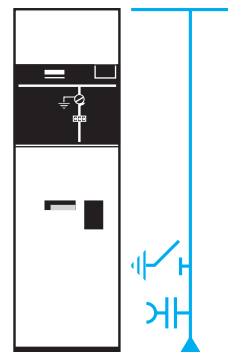
Célula de entrada ou saída de cabos GAM (500 mm)
