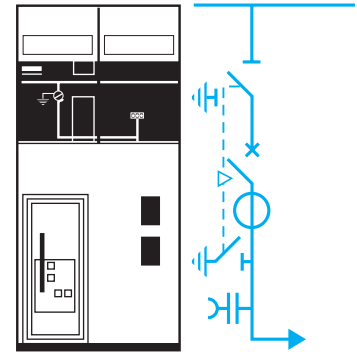
Disjuntor desconectável simples seccionamento à direita DMVL-D (750 mm)
